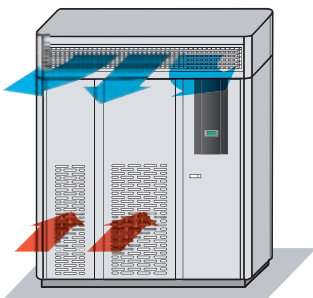
带有风帽从前面进风的上送风机组
