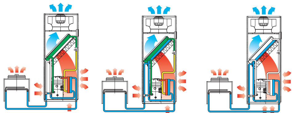
Fig. A 单一机械制冷
